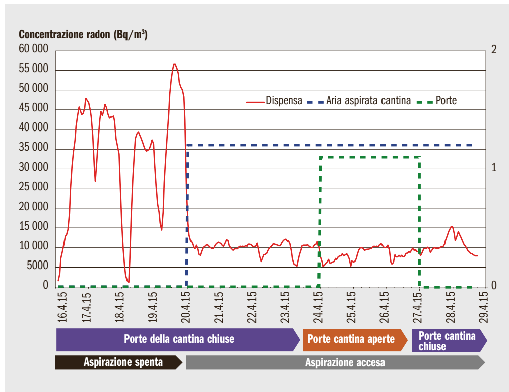
Figura 6.83: Il ventilatore installato in cantina riduce le concentrazioni fino a valori che si situano tra gli 8000 Bq/m 3 e i 12000 Bq/m 3 , concentrazioni che risultano essere ancora troppo elevate.
