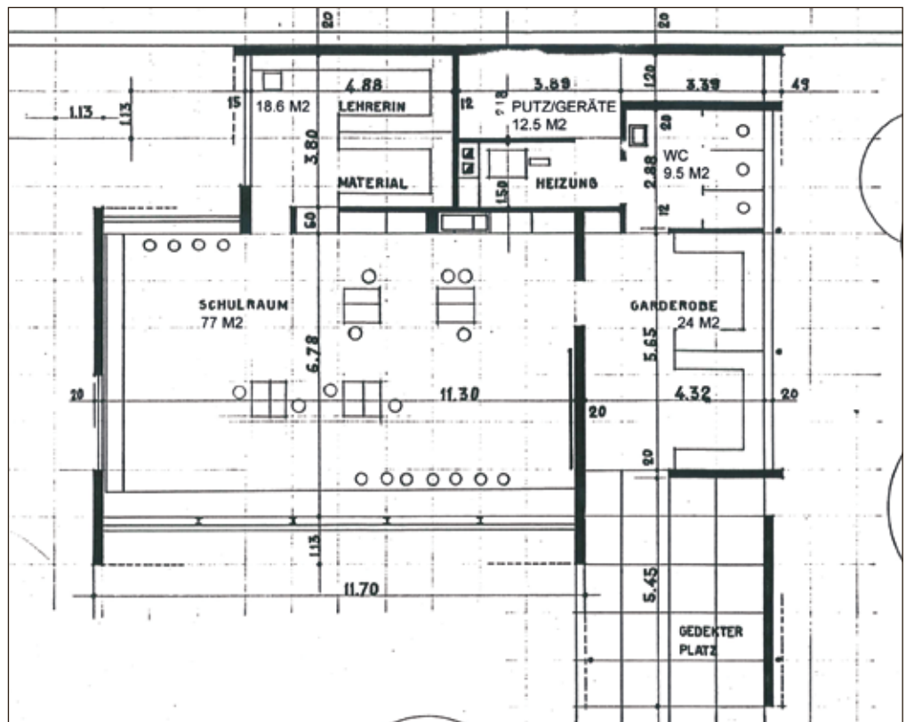
Figura 6.64: Per la protezione dal radon, la superficie della sala principale di 77 m² è stata una sfida.
