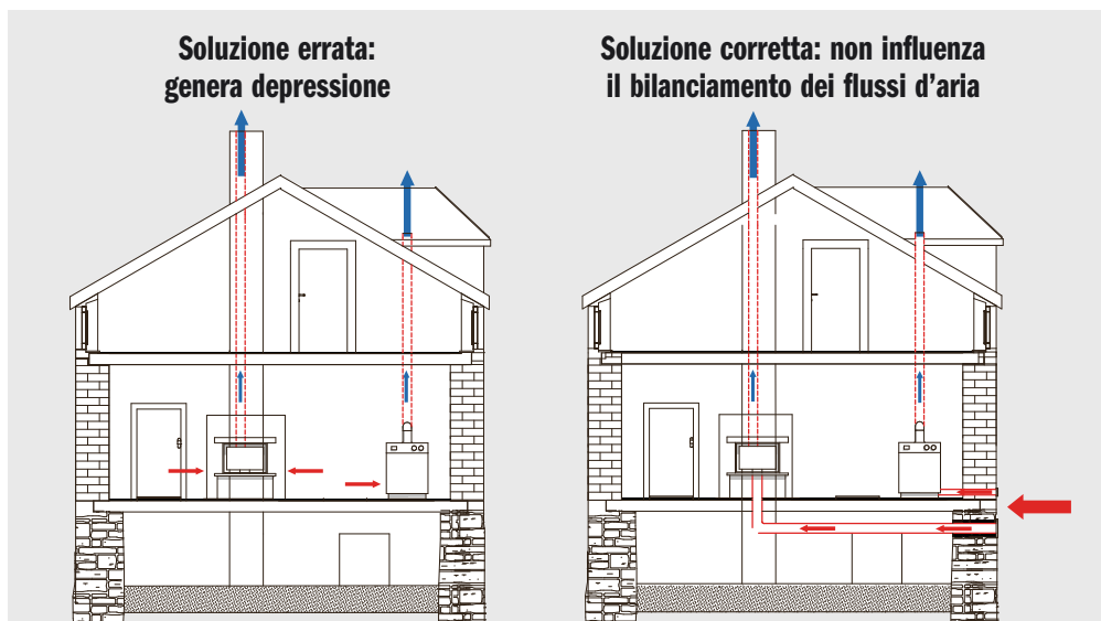
Figura 5.6: Grazie ad un'adduzione dall'esterno dell'aria comburente del camino o della cappa della cucina si evita la creazione di una depressione all'interno dei locali abitativi (Fonte: SMUL).
