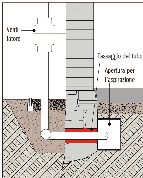
Figura 5.20: Pozzo radon (Fonte: SMUL).
