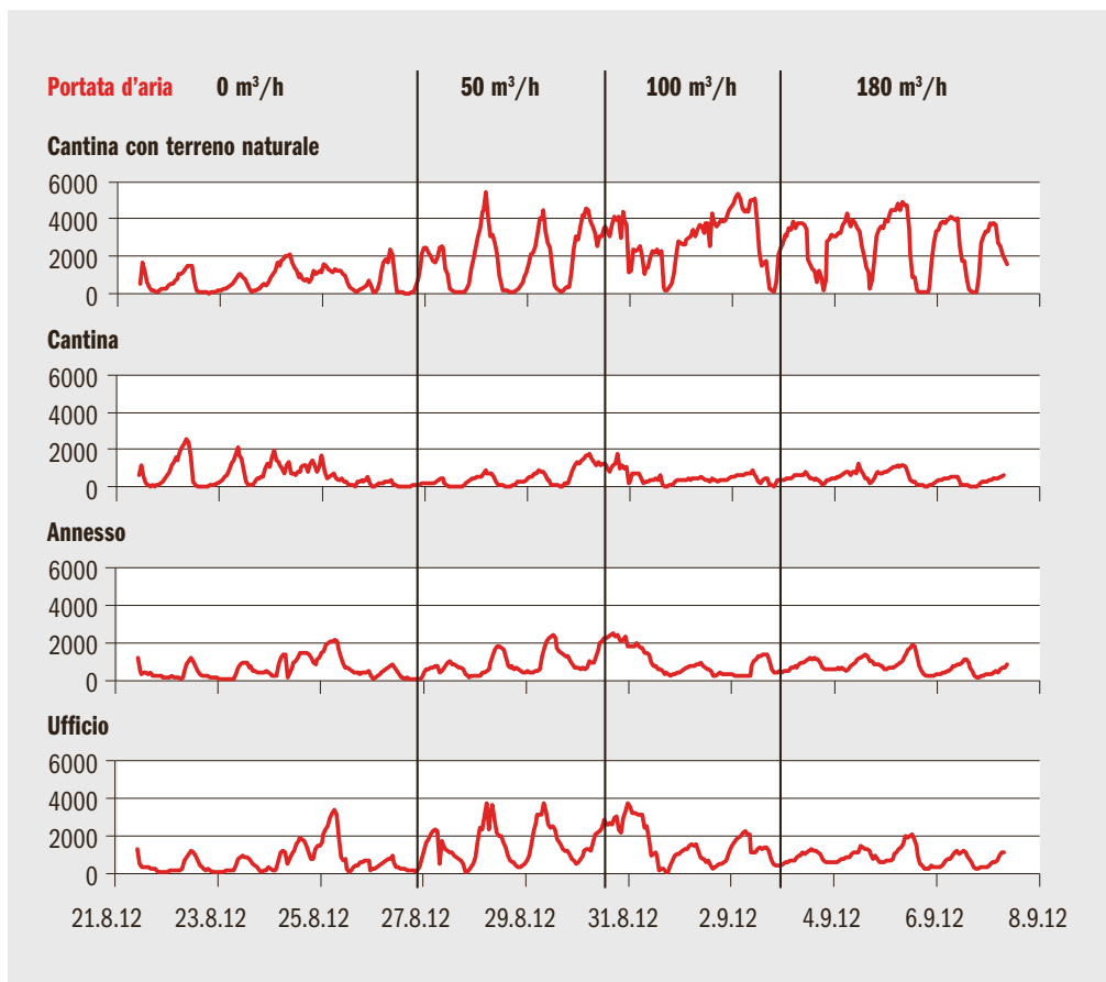
Figura 6.38: La ventilazione della cantina ha mostrato un ridotto effetto sulle concentrazioni radon (nonostante un aumento del volume ventilato che è ora pari a 180 m 3 /h). Le dinamiche termiche invece sono chiaramente visibili. I valori radon fluttuano fortemente a seconda della radiazione solare e della temperatura ambientale.
