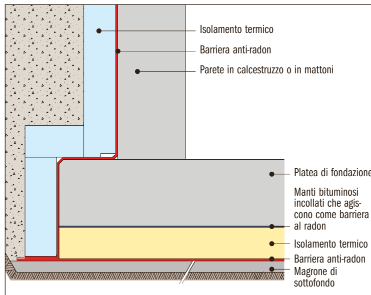
Figura 4.7: Nuova costruzione con isolamento perimetrale e platea di fondazione con scantinato (Fonte: Dow Building Solutions).
